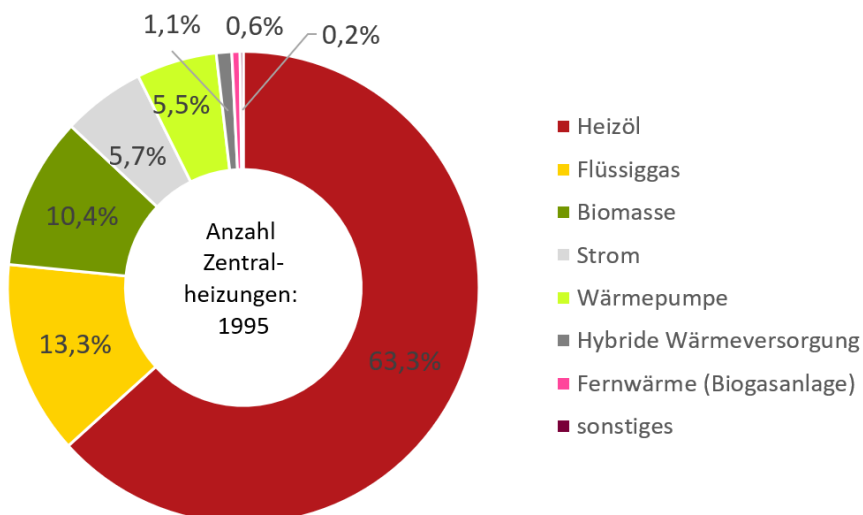
Abbildung 10: Anteil der Hauptwärmequelle nach Heizart/Energieträger
