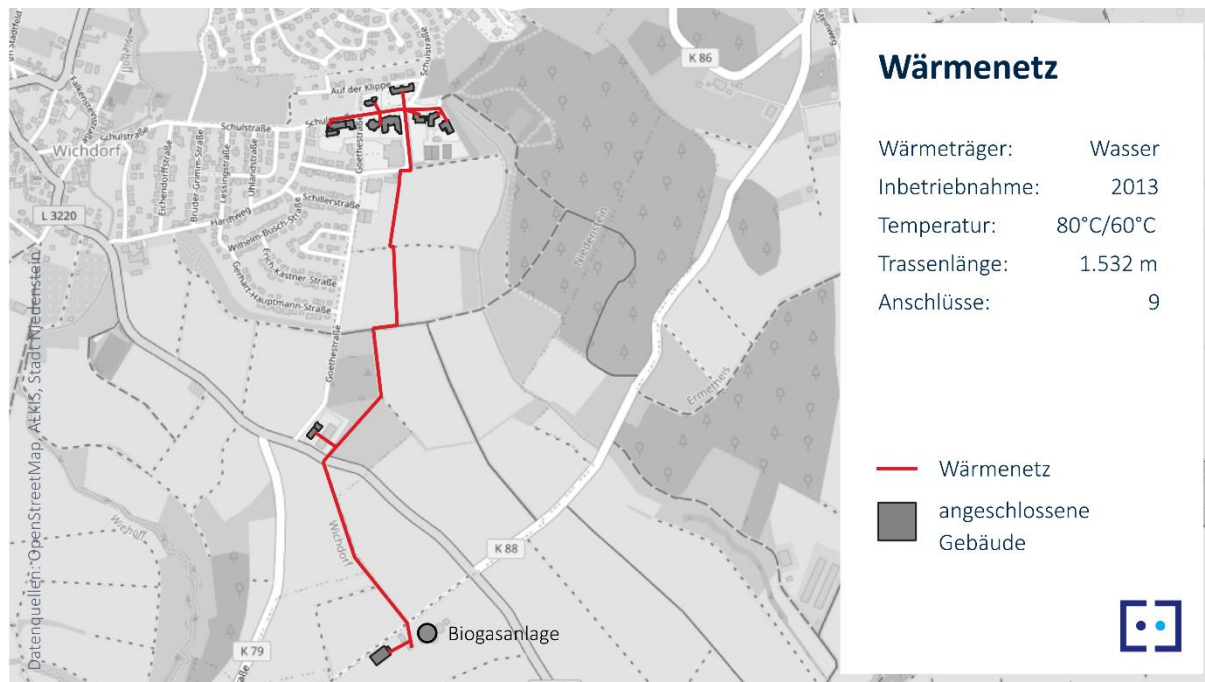
Abbildung 8: Wärmenetz Wichdorf/Niedenstein
