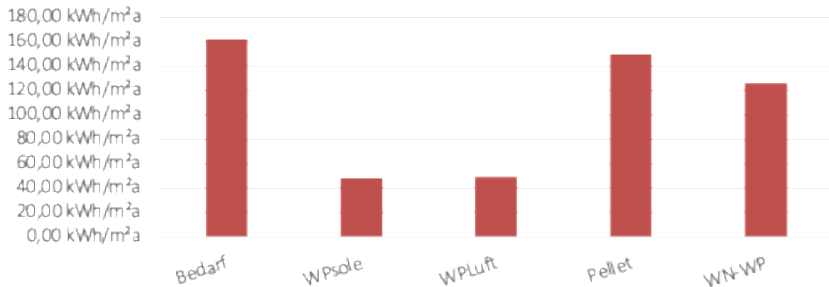
Abbildung 29: Spezifischer Endenergiebedarf für die Wärme in kWh pro Jahr
